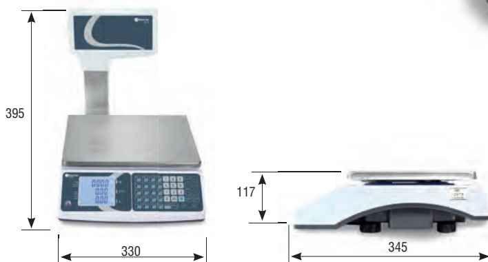
Dimensões (mm)
